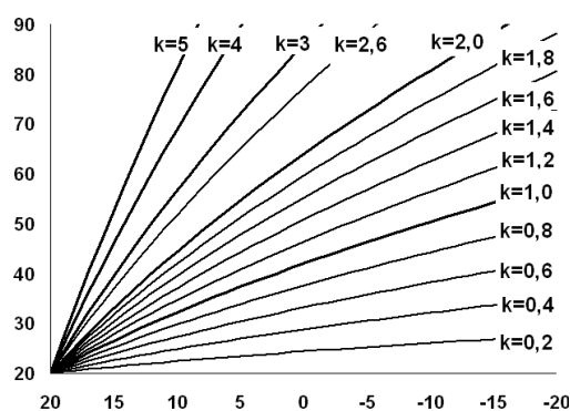
Figura 5. Curve equi-termiche
